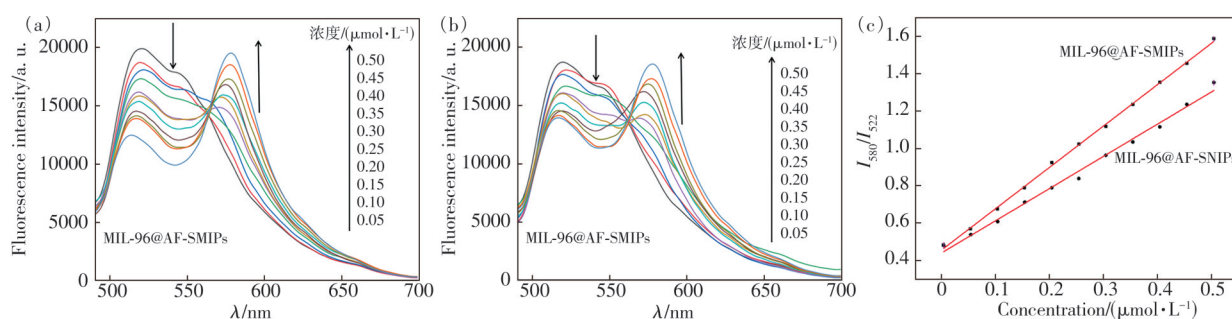
图5 MIL-96@AF-SMIPs(a)和MIL-96@AF-SNIPs(b)随罗丹明B浓度变化的荧光光谱;(c)MIL-96@AF-SMIPs和MIL-96@AF-SNIPs的 I_{580}/I_{522} 随罗丹明B浓度变化的线性关系
