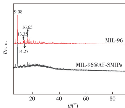
图2 MIL-96 和 MIL-96@AF-SMIPs 的 XRD 图
